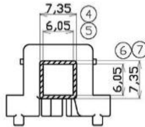
截面 A-A
